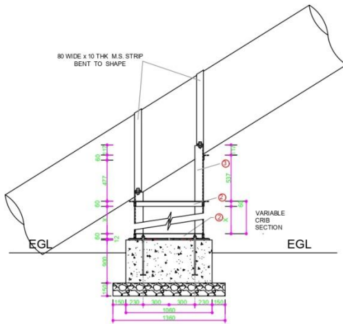
RIGHT FACE ELEVATION
